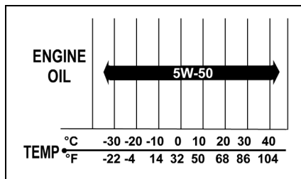
ÖLTABELLE
